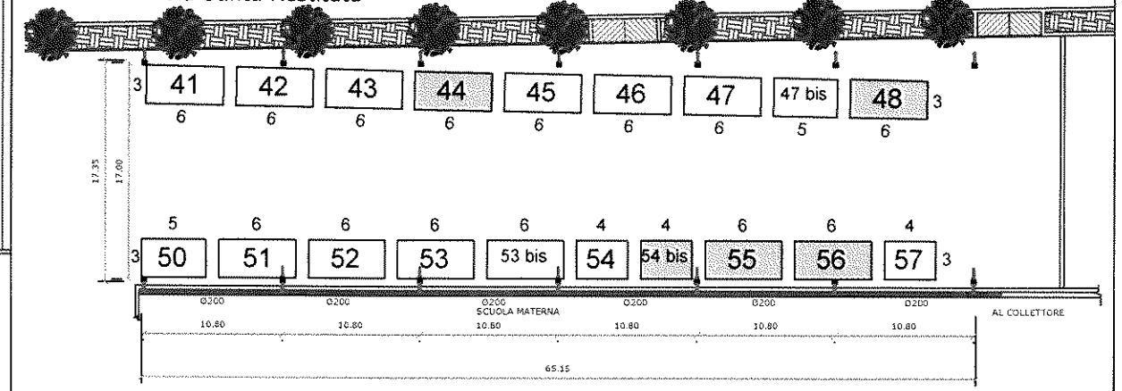
PIANTA TETTOIA B Via Santa Restituta
